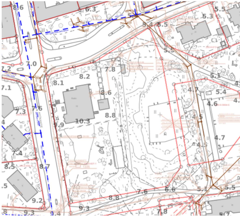
Kuva: Johtokartta Hovinsaaren koulun tontin kohdalla.
